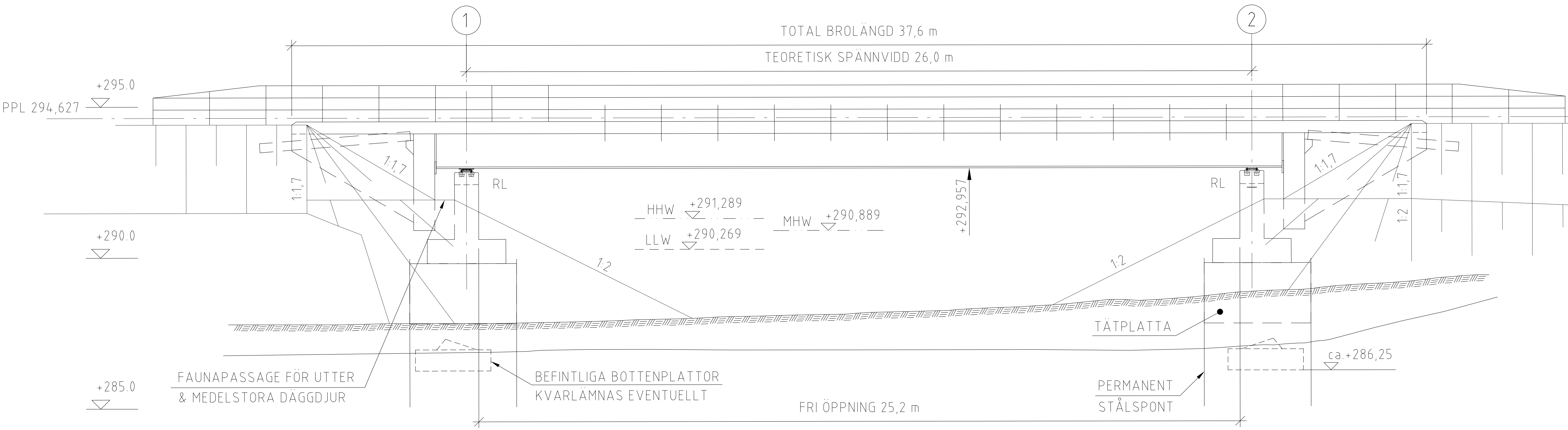
ELEVATION 1:100
